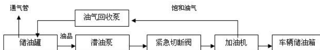
图 2.2-3 汽油加油工艺流程示意简图
