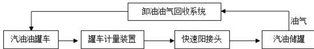
图 2.2-1 汽油卸油工艺流程示意简图
