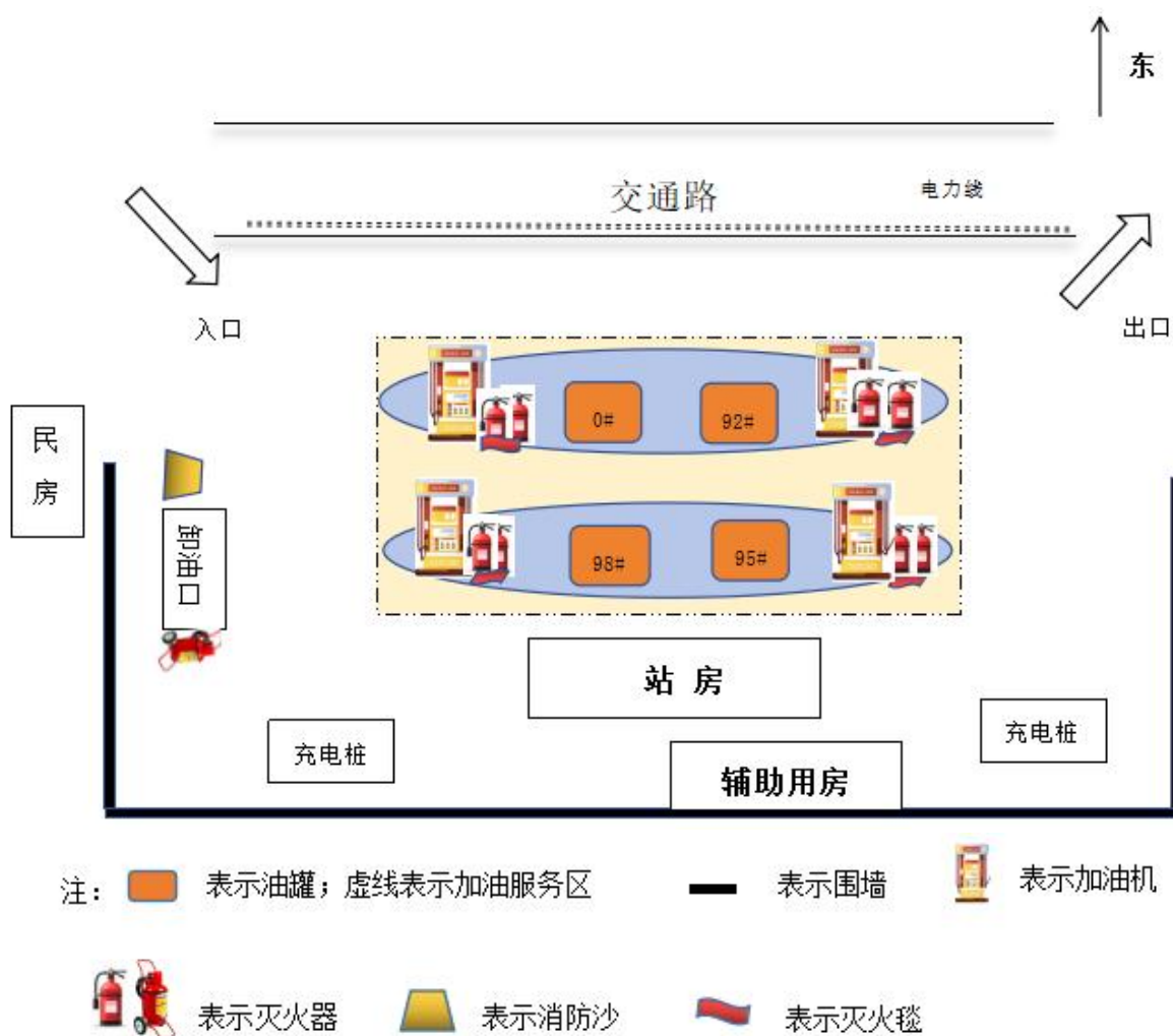
图 2.3-1 加油站平面布置简图
