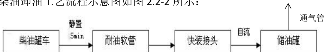
图 2.2-2 柴油卸油工艺流程示意简图
