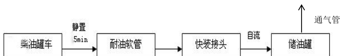
图 2.2-2 柴油卸油工艺流程示意简图
