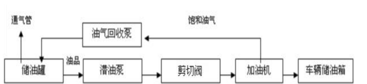
图 2.2-3 汽油加油工艺流程示意简图
