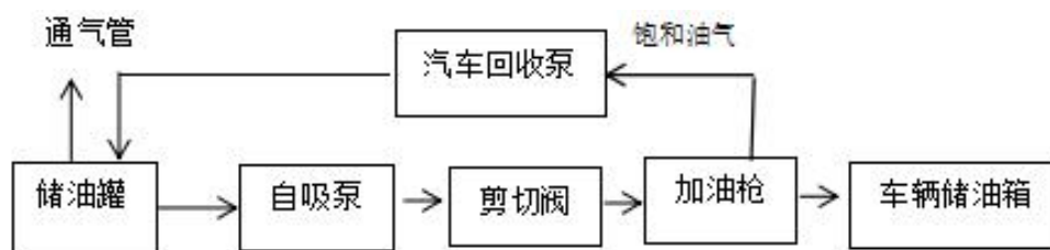
图 2.2-3 汽油加油工艺流程示意简图
