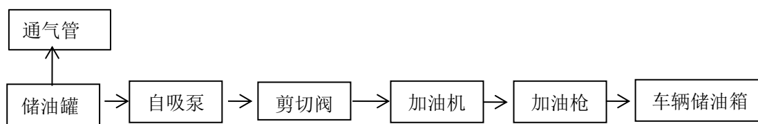
图 2.2-4 柴油加油工艺流程示意简图
