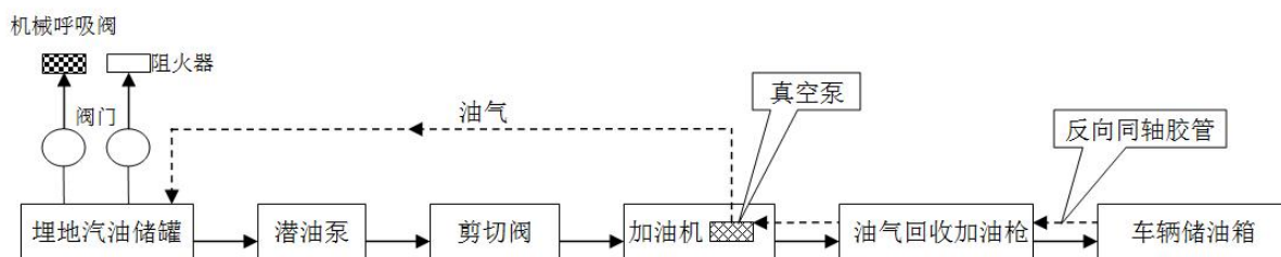
图 2.2-3 汽油加油工艺流程示意简图
