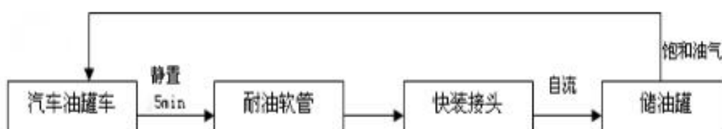
图 2.2-1 汽油卸油工艺流程示意简图
