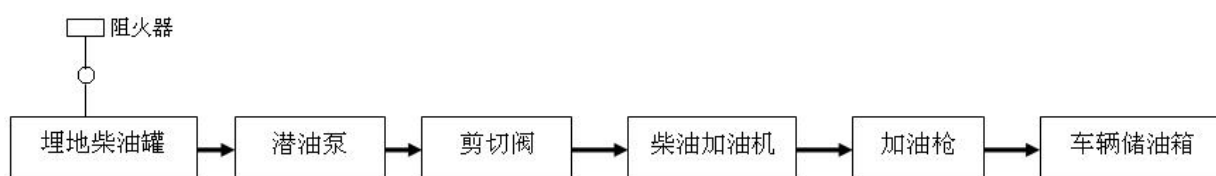
图 2.2-4 柴油加油工艺流程示意简图
