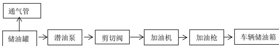
图 2.2-4 柴油加油工艺流程示意简图
