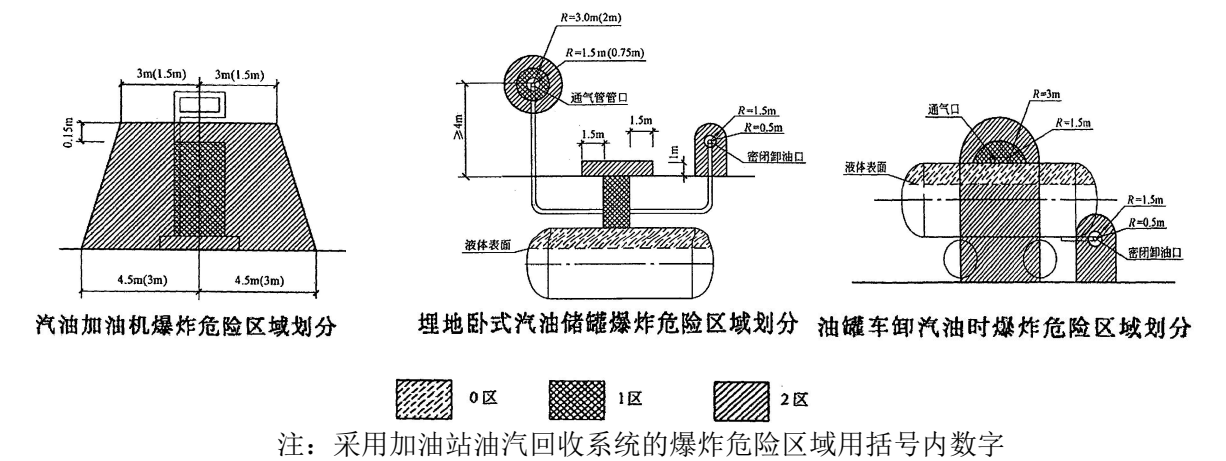
图 3.5.10-1 加油机、埋地汽油罐、卸油口爆炸危险区域划分图
