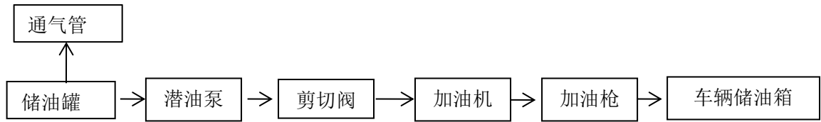
图 2.2-4 柴油加油工艺流程示意简图
