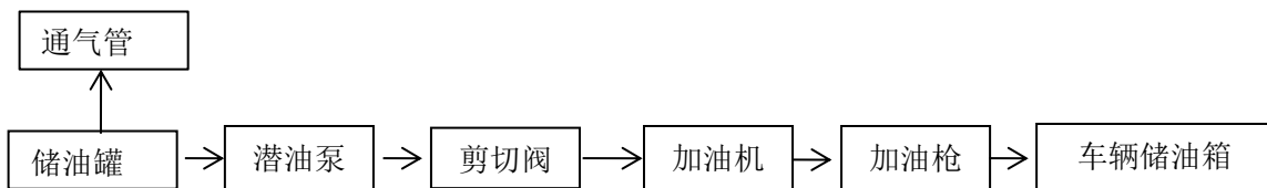
图 2.2.2-4 柴油加油工艺流程示意简图
