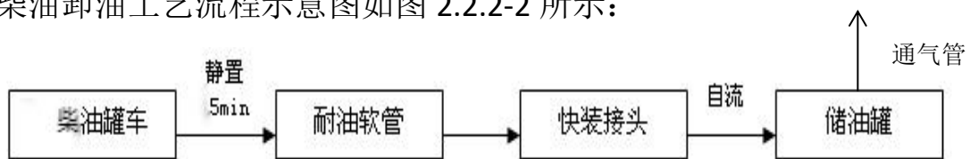
图 2.2.2-2 柴油卸油工艺流程示意简图
